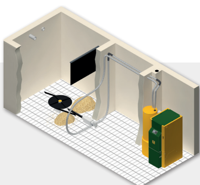
MEŠALNI DISK KWB PLUS ZA PELETE S SESALNIM TRANSPORTOM
