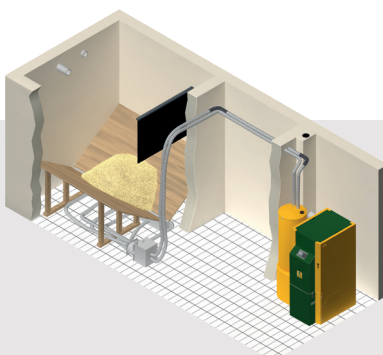
ODJEMNE SONDE KWB ALI 1-TOČKOVNA ODJEMNA SONDA S SESALNIM TRANSPORTOM
