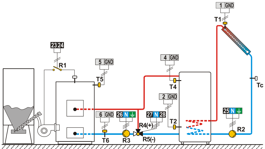
Shema 262b (SGC67) - Kotel na pelete, hranilnik toplote, solarni kolektorji.
