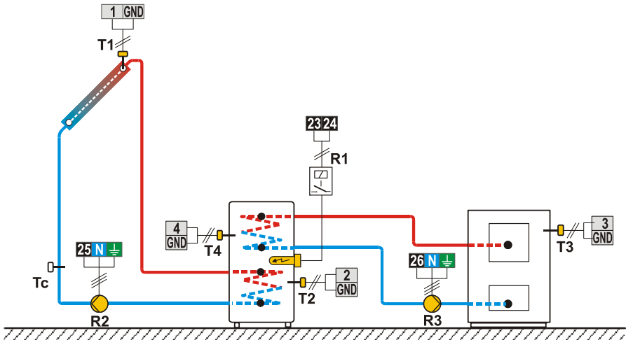
Shema 231d (SGC36, SGC67) - Solarni kolektorji, grelnik sanitarne vode, kotel na trdo kurivo, dogrevanje z elektriko.
