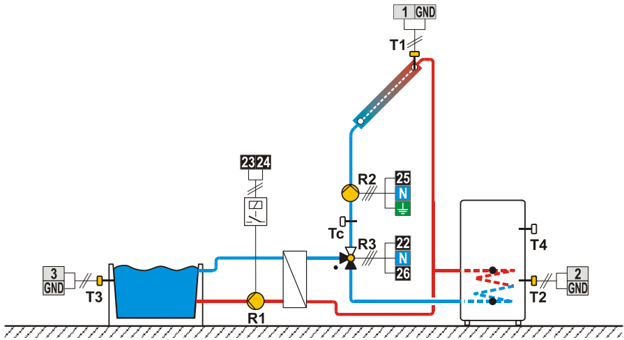
Shema 234 (SGC36, SGC67) - Solarni kolektorji, grelnik sanitarne vode, bazen, preklp.
