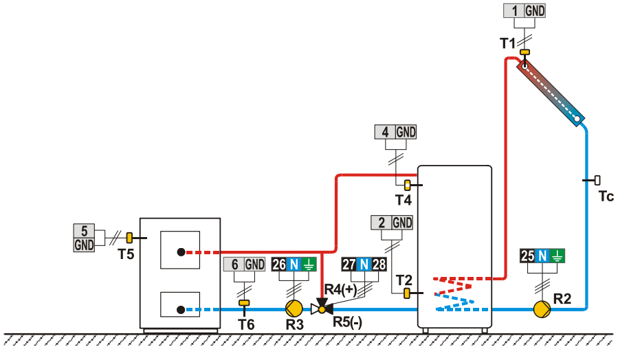
Shema 262 (SGC67) - Kotel na trdo gorivo, hranilnik toplote, solarni kolektorji.
