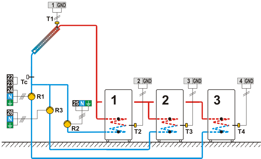
Shema 247 (SGC36, SGC67) - Solarni kolektorji, trije grelniki sanitarne vode, tri črpalke.
