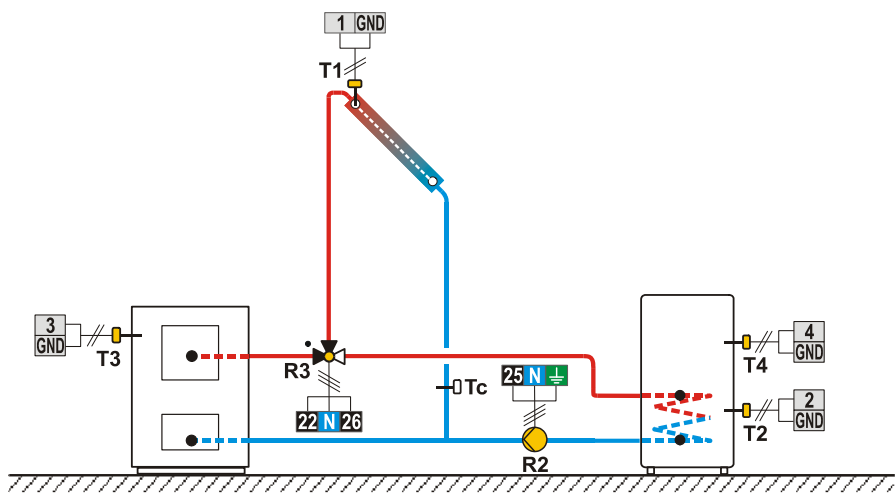
Shema 243 (SGC36, SGC67) - Kotel na trdo kurivo, solarni kolektorji, grelnik sanitarne vode, preklap.
