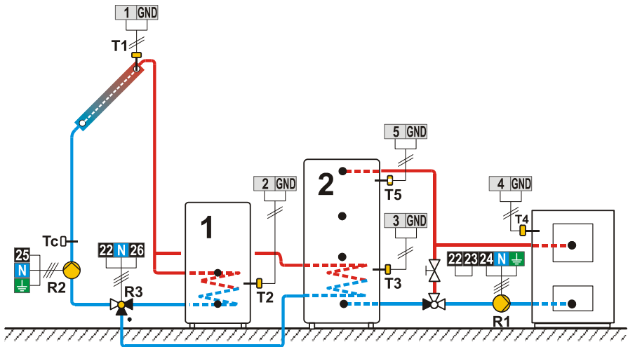
Shema 232b (SGC36, SGC67) - Solarni kolektorji, grelnik sanitarne vode, hranilnik toplote, preklap, kotel na trdo kurivo.
