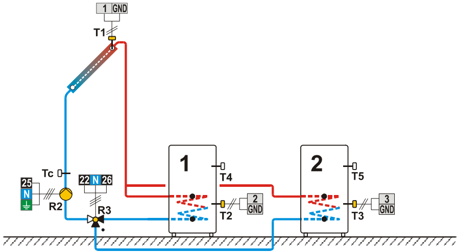
Shema 232 (SGC36, SGC67) - Solarni kolektorji, dva grelnika sanitarne vode, preklap.
