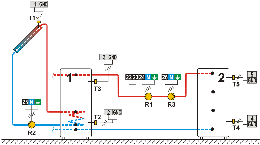
Shema 246b (SGC36, SGC67) - Reverzibilni prenos toplote med glavnim in pomožnim hranilnikom toplote, dve črpalke.
