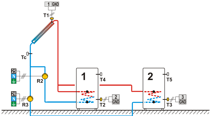
Shema 233 (SGC36, SGC67) - Solarni kolektorji, dva grelnika sanitarne vode, dve črpalci.
