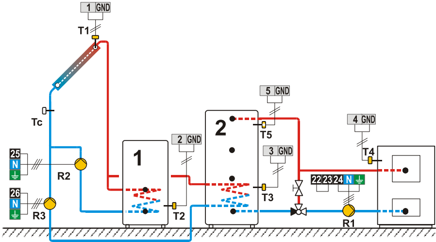
Shema 233b (SGC36, SGC67) - Solarni kolektorji, grelnik sanitarne vode, hranilnik toplote, kotel na trdo kurivo.
