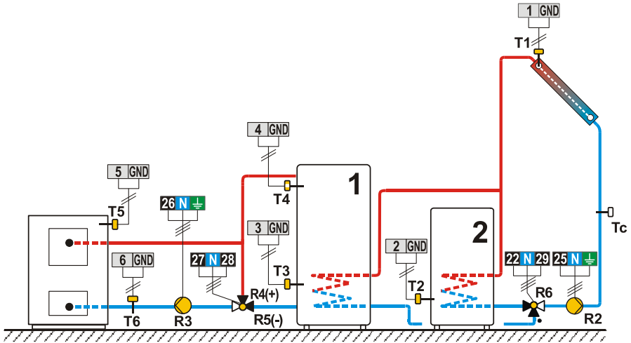
Shema 263 (SGC67) - Kotel na trdo gorivo, hranilnik toplote, grelnik sanitarne vode, solarni kolektorji.
