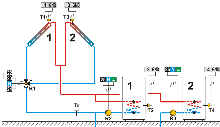
Shema 248c (SGC36, SGC67) - Solarni kolektorji vzhod - zahod, prekllop, dva grelnika sanitarna vode, dve črpalčki.
