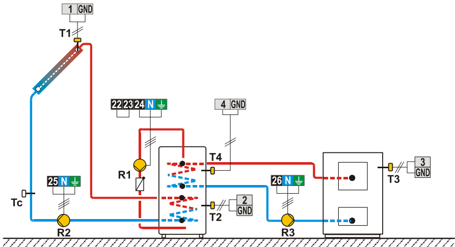
Shema 241 (SGC36, SGC67) - Solarni kolektorji, grelnik sanitarne vode, kotel na trdo kurivo.
