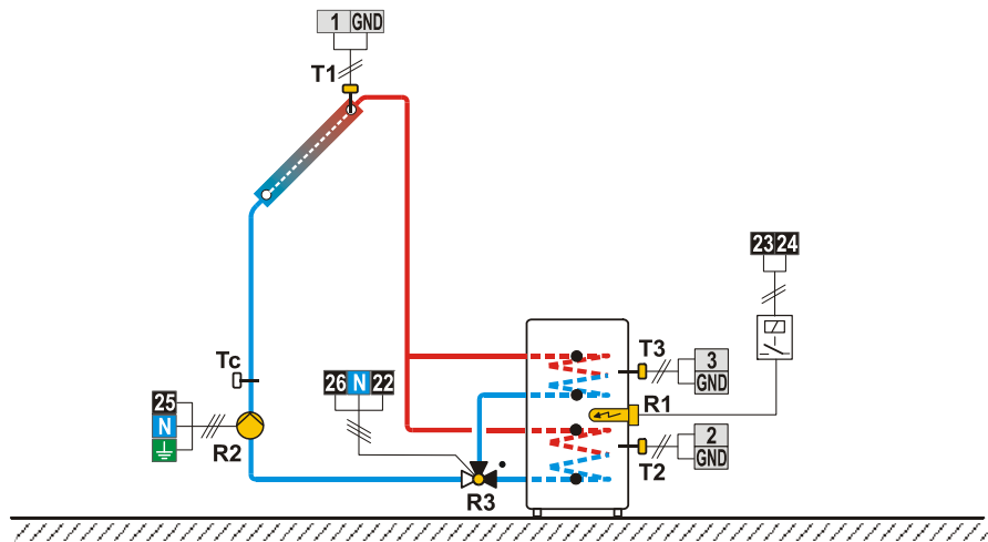
Shema 239 (SGC36, SGC67) - Solarni kolektorji, grelnik sanitarne vode, preklap zgoraj/spodaj, dogrevanje z elektriko.
