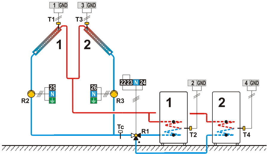
Shema 248 (SGC36, SGC67) - Solarni kolektorji vzhod - zahod, dve črpalke, dva grelnika sanitarne vode, prekllop.
