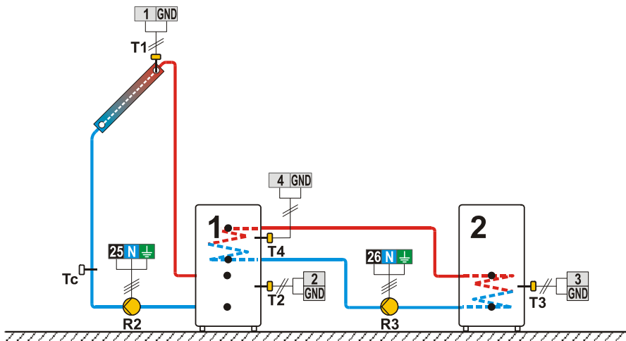
Shema 237 (SGC36, SGC67) - Solarni kolektorji, dva grelnika sanitarne vode, prenos toplote v 2. grelnik sanitarne vode.
