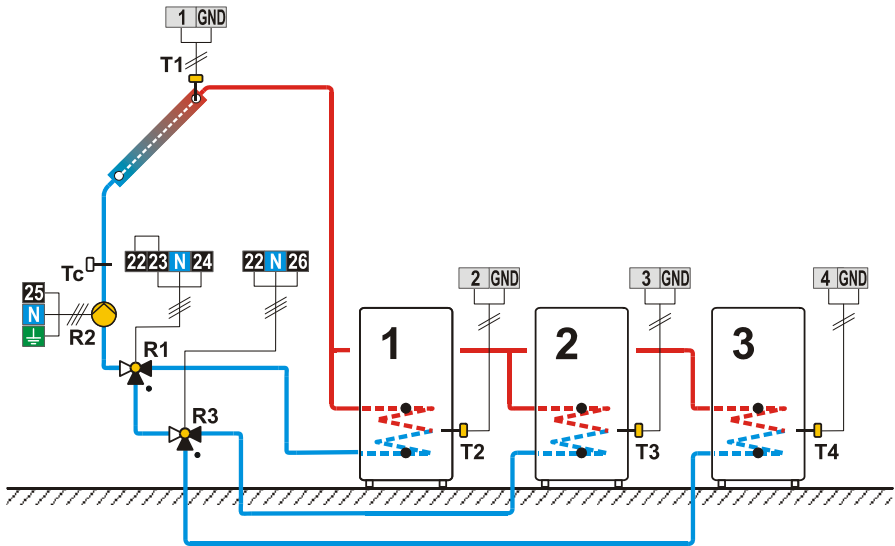
Shema 247b (SGC36, SGC67) - Solarni kolektorji, trije grelniki sanitarne vode, prekllop.
