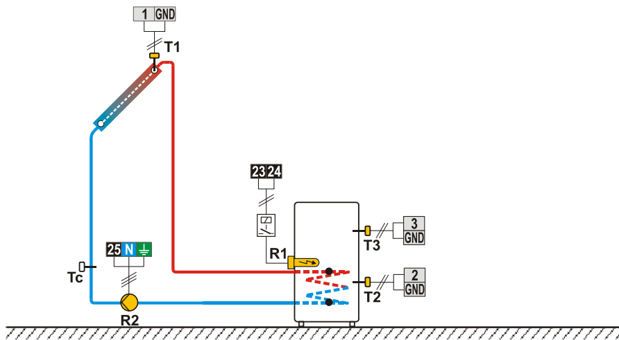
Shema 214 (SGC26, SGC36, SGC67) - Solarni kolektorji, grelnik sanitarne vode, dogrevanje z elektriko.
