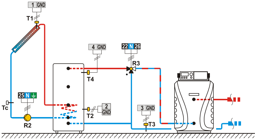
Shema 240 (SGC36, SGC67) - Solarni kolektorji, podpora ogrevanja s hranilnikom toplote.
