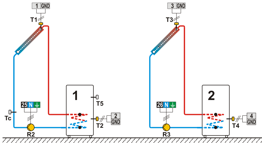
Shema 238 (SGC36, SGC67) - Solarni kolektorji, grelnik sanitarne vode, dva ločena kroga.
