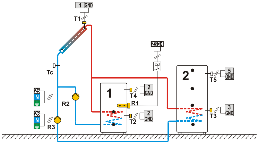
Shema 233c (SGC36, SGC67) - Solarni kolektorji, grelnik sanitarne vode, hranilnik toplote, električni grelec.
