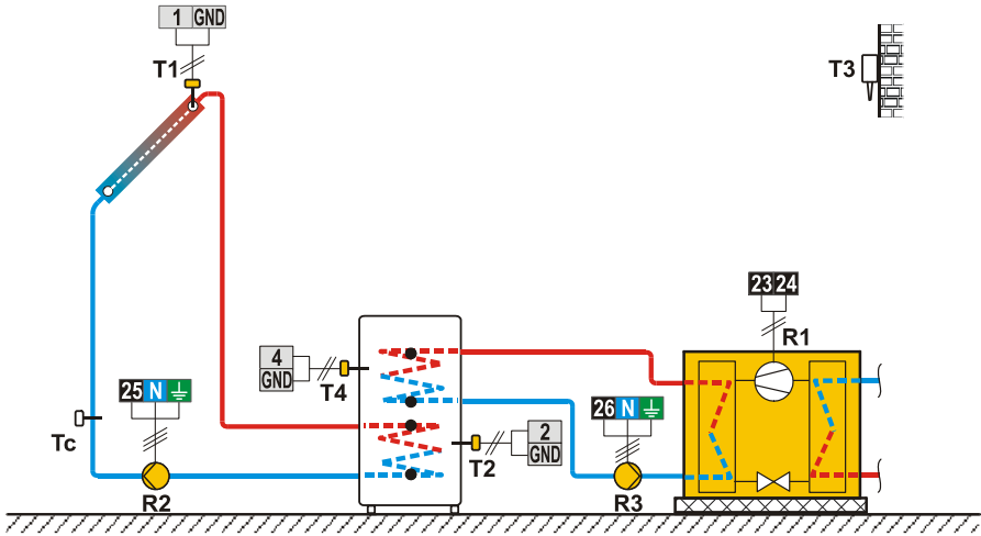
Shema 231c (SGC36, SGC67) - Solarni kolektorji, grelnik sanitarne vode, toplotna črpalka.
