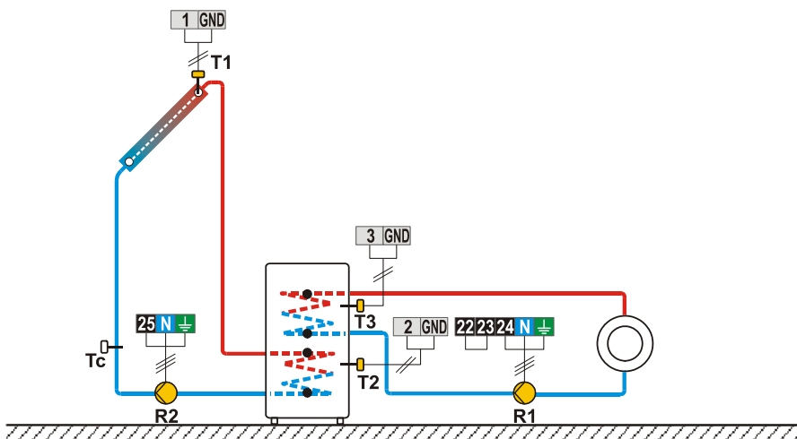
Shema 216 (SGC26, SGC36, SGC67) - Solarni kolektorji, grelnik sanitarne vode, odvzem presežka toplote.
