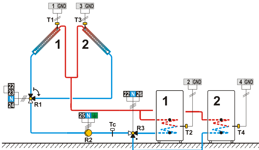
Shema 248b (SGC36, SGC67) - Solarni kolektorji vzhod - zahod, prekllop, dva grelnika sanitarna vode, prekllop.
