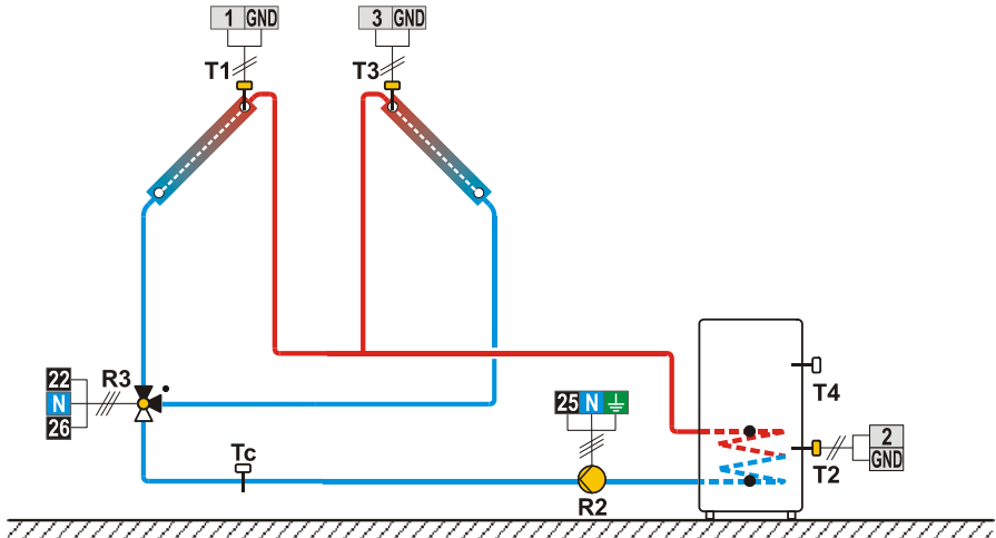
Shema 235 (SGC36, SGC67) - Solarni kolektorji vzhod - zahod, grelnik sanitarne vode, preklp.
