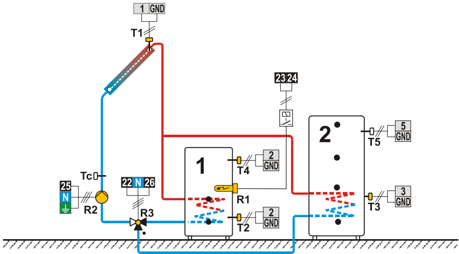
Shema 232c (SGC36, SGC67) - Solarni kolektorji, grelnik sanitarne vode, hranilnik toplote, preklop, električni grelec.
