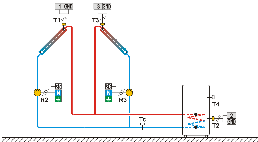
Shema 236 (SGC36, SGC67) - Solarni kolektorji vzhod - zahod, grelnik sanitarne vode, dve črpalčki.
