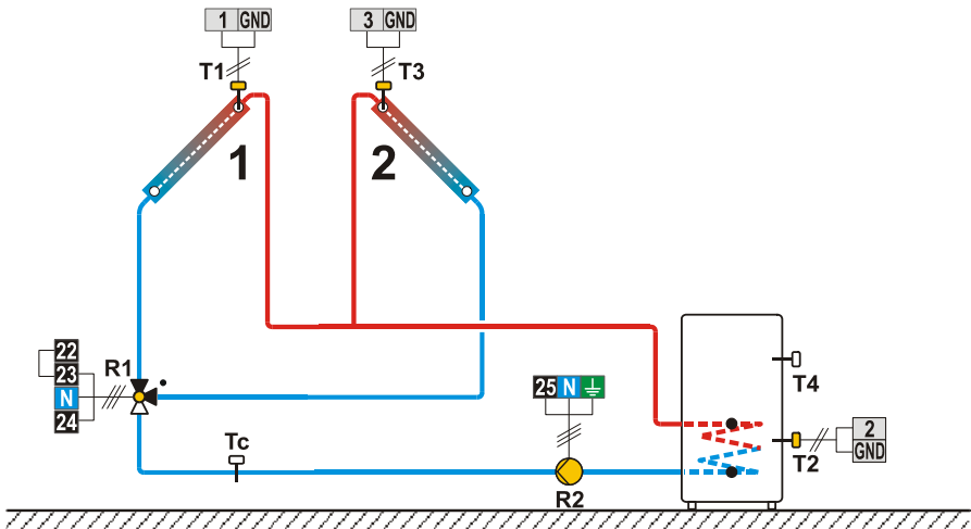
Shema 223 (SGC26, SGC36, SGC67) - Solarni kolektorji vzhod - zahod, grelnik sanitarne vode, prekllop.
