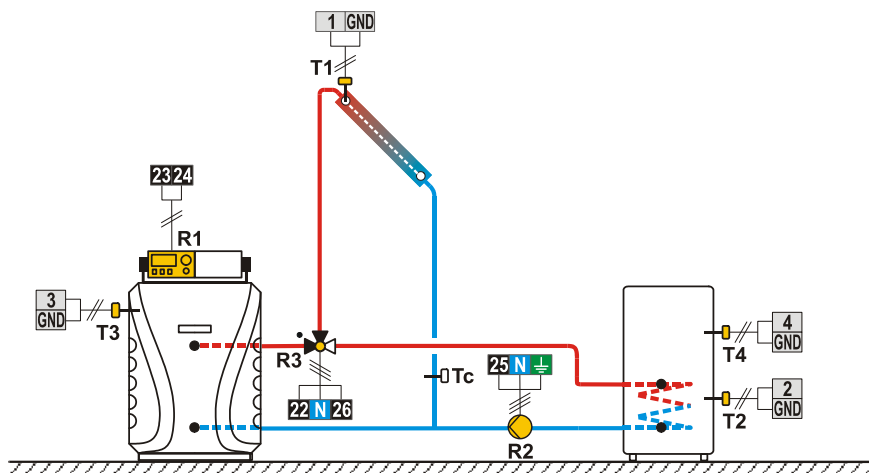
Shema 243b (SGC36, SGC67) - Kotel na tekoče kurivo, solarni kolektorji, grelnik sanitarne vode, preklap.
