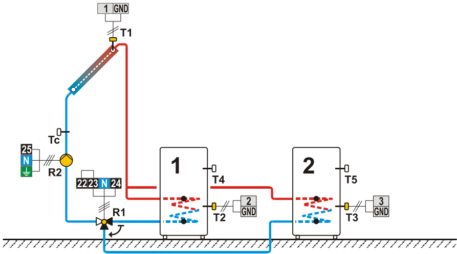
Shema 222 (SGC26, SGC36, SGC67) - Solarni kolektorji, dva grelnika sanitarne vode, prekllop.
